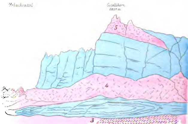
Fig. 3. Die oberen 3 Gneisskeile am Gstellhorn (3, 4, 5)
